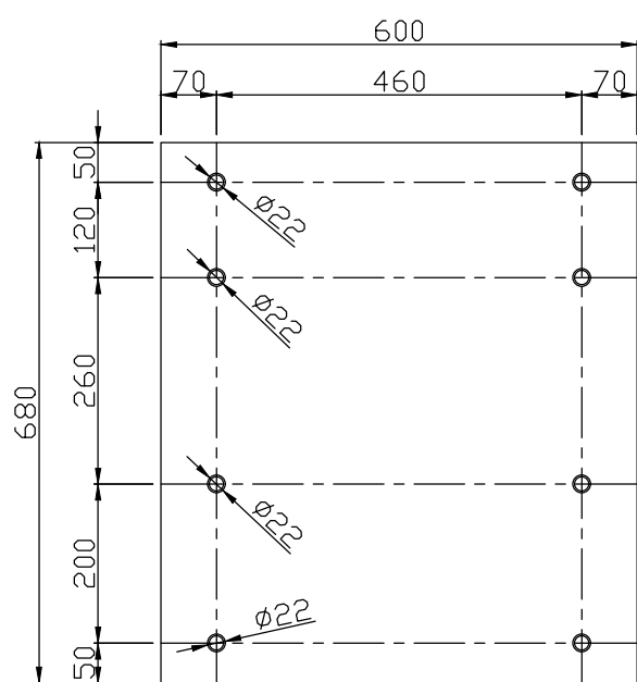
CHAPA DE LIGAÇÃO CHAPA # 1/2" QUANTIDADE: 02 PÇS
