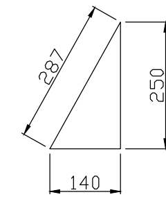
PEÇA A CHAPA # 5/8" QUANTIDADE : 08 PÇS
