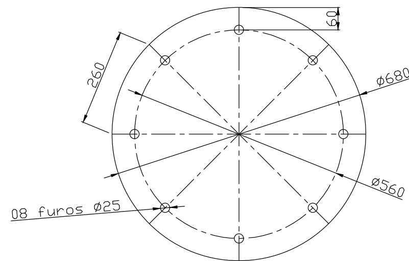
CHAPA GABARITO CHAPA # 14" QUANTIDADE: 01 PÇ
