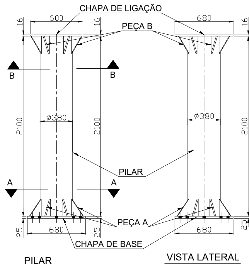
PILAR VISTA DA FRENTE QUANTIDADE: 01 PÇ
